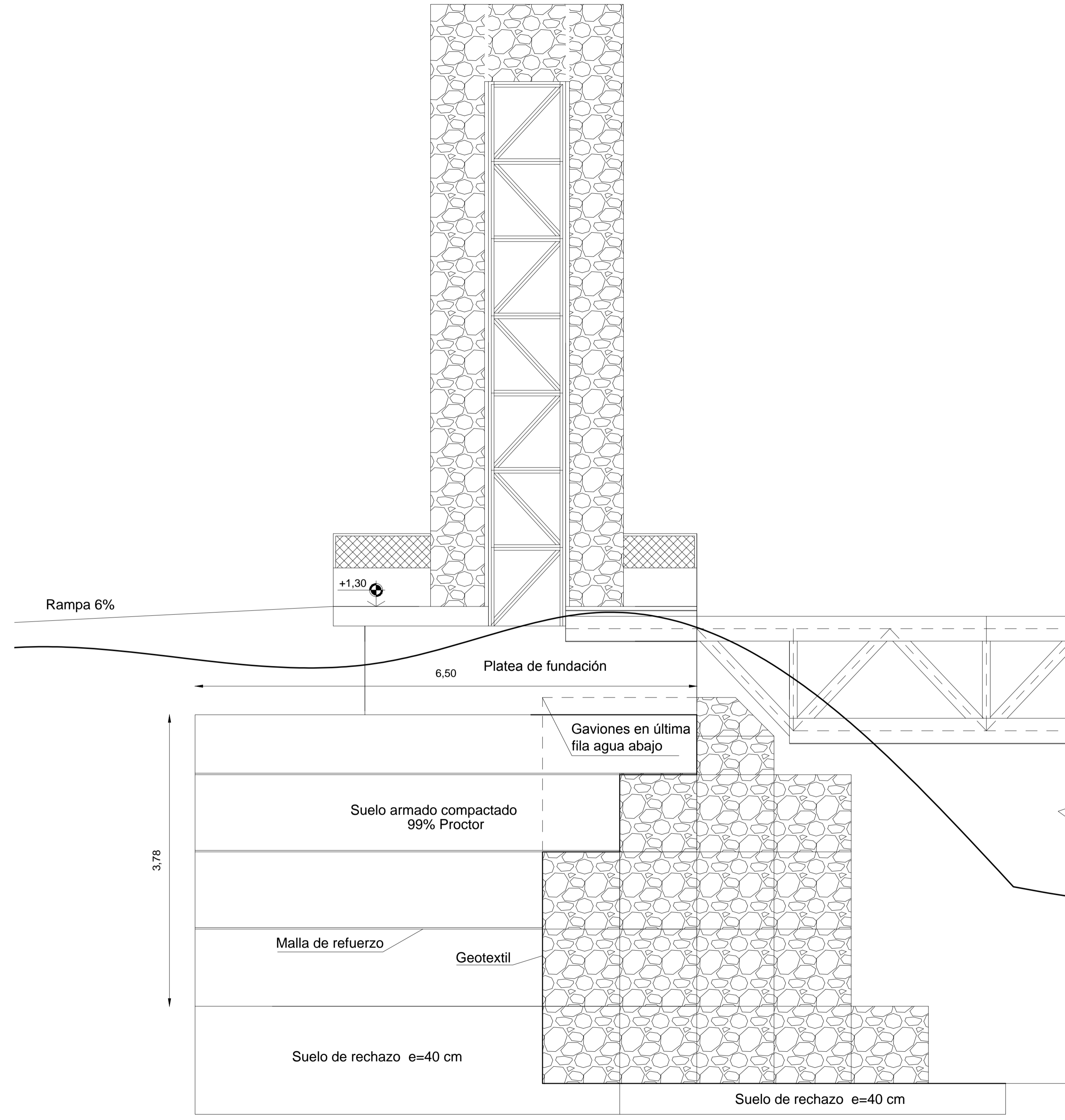
CORTE 2 - VISTA LATERAL MURO DE CONTENCIÓN (Sin platea de fundación)
