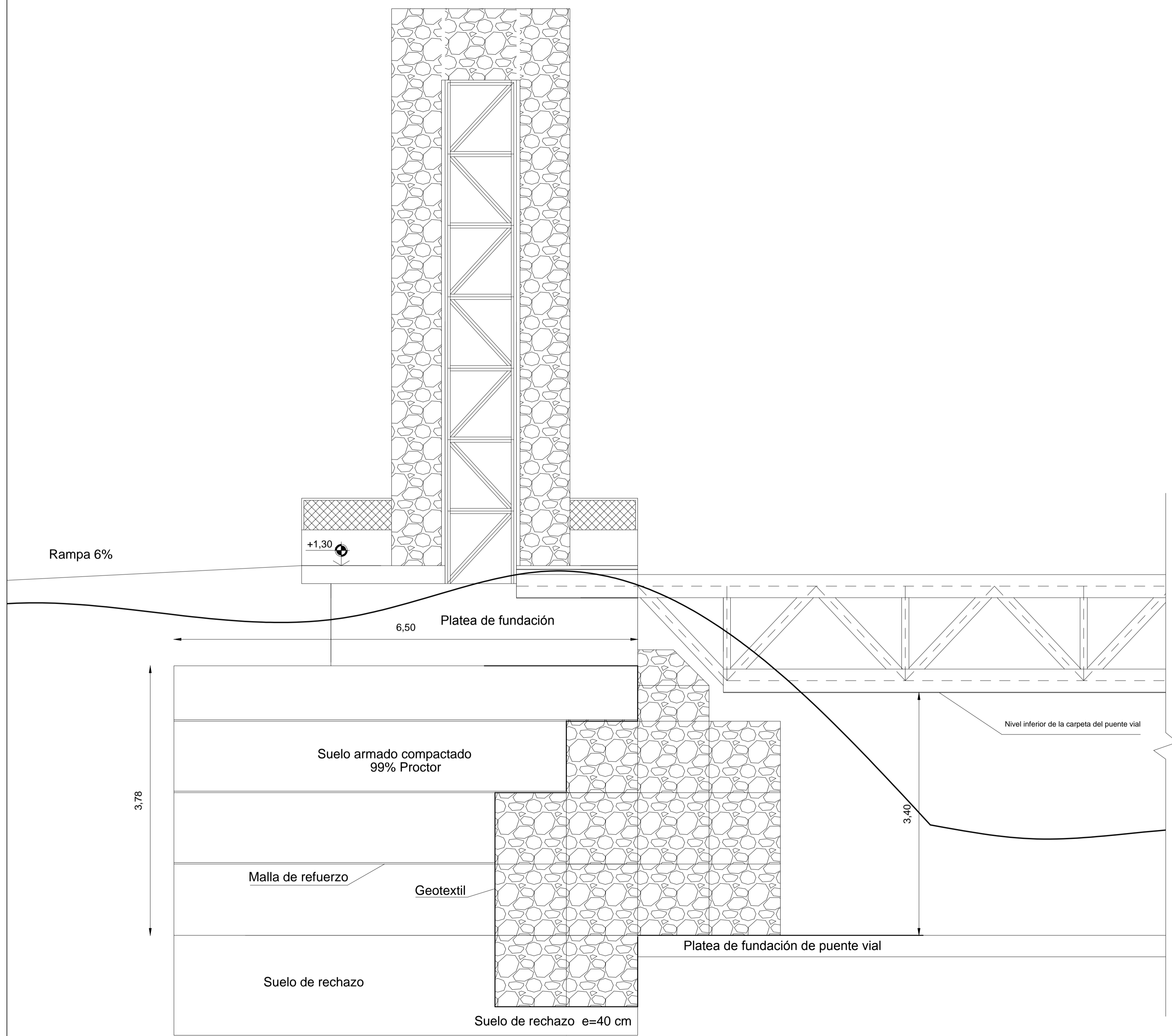
CORTE 1- VISTA LATERAL MURO DE CONTENCIÓN (Con platea de fundación)
