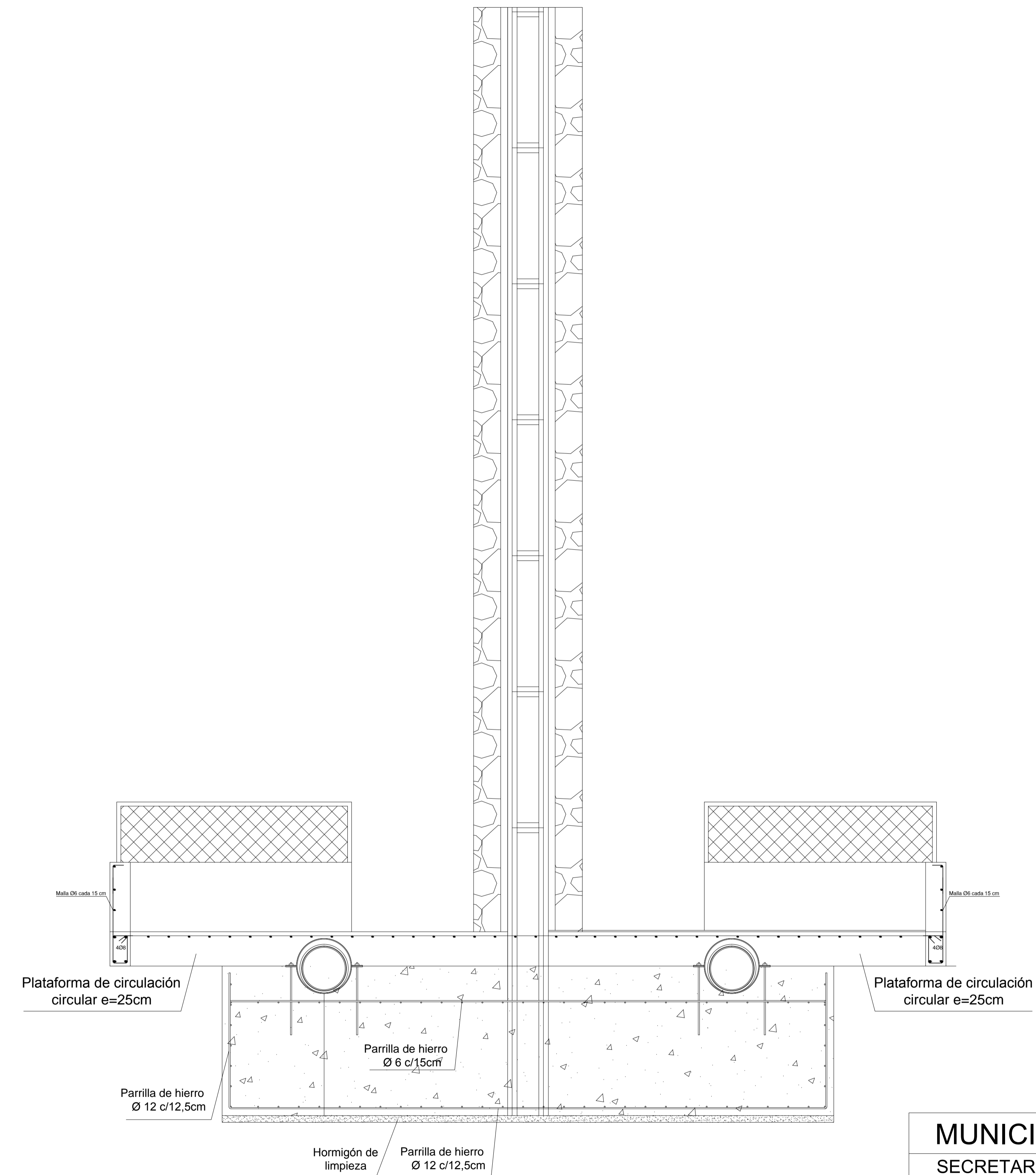
CORTE B
