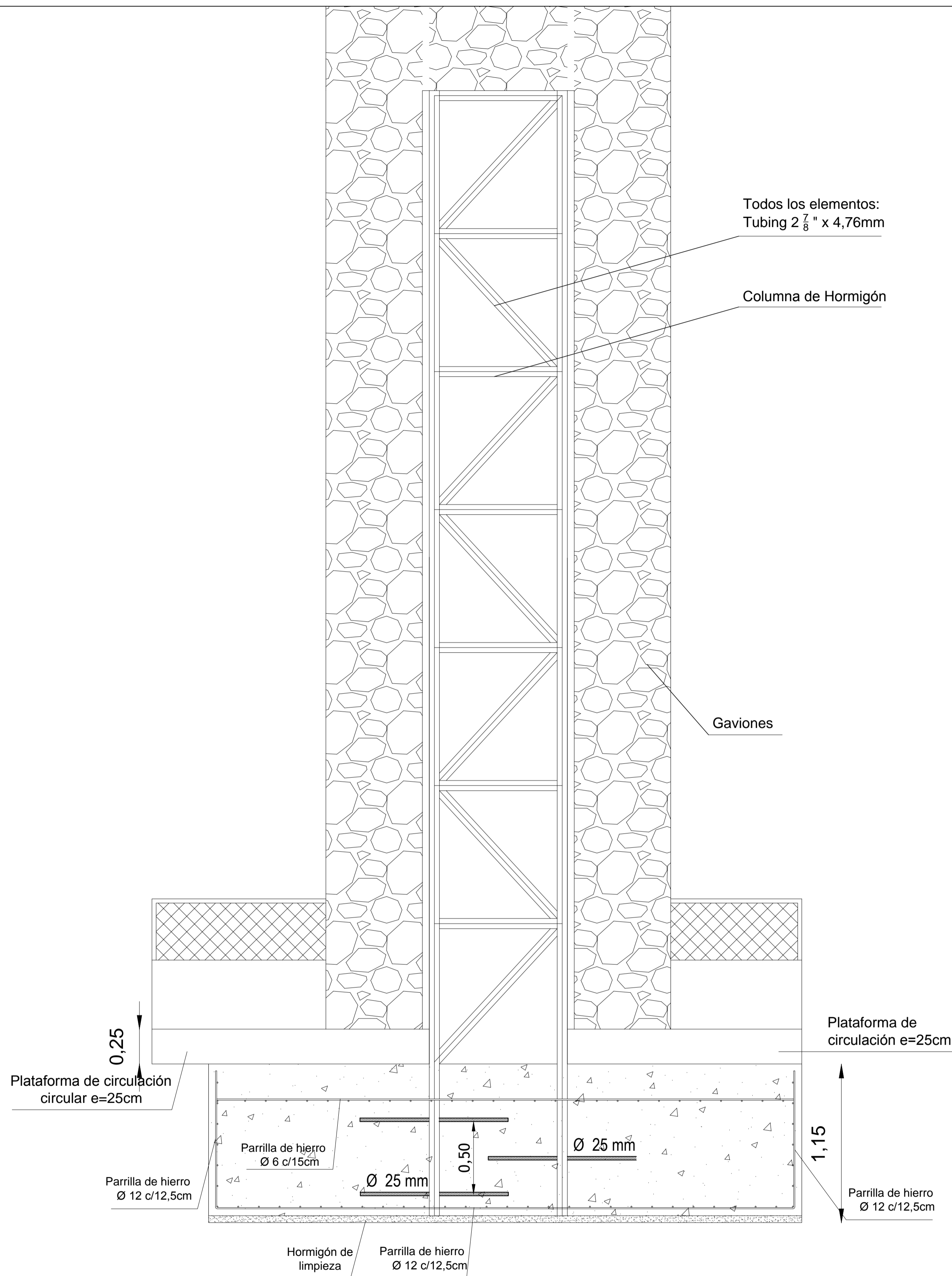
CORTE A
