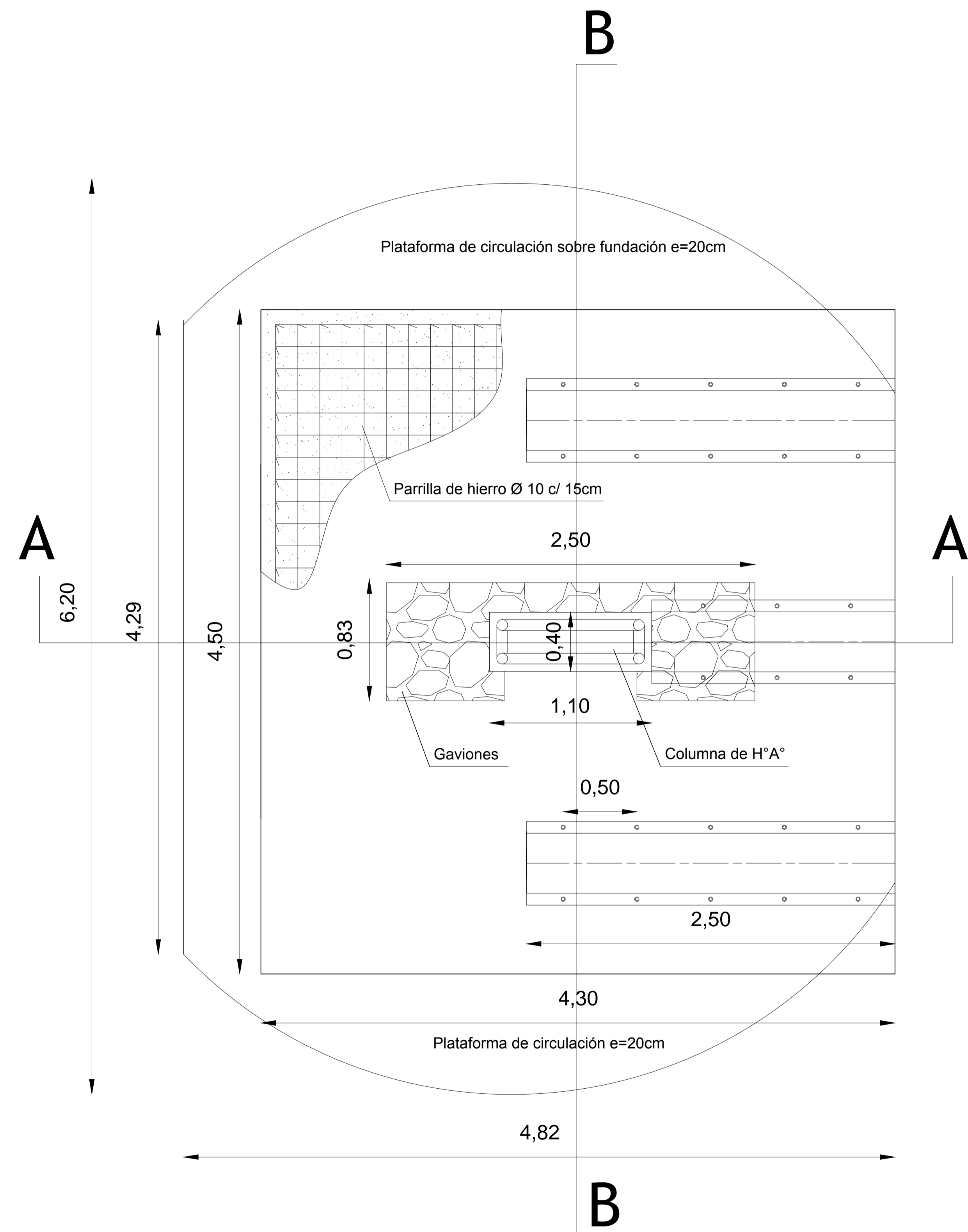
PLANTA
