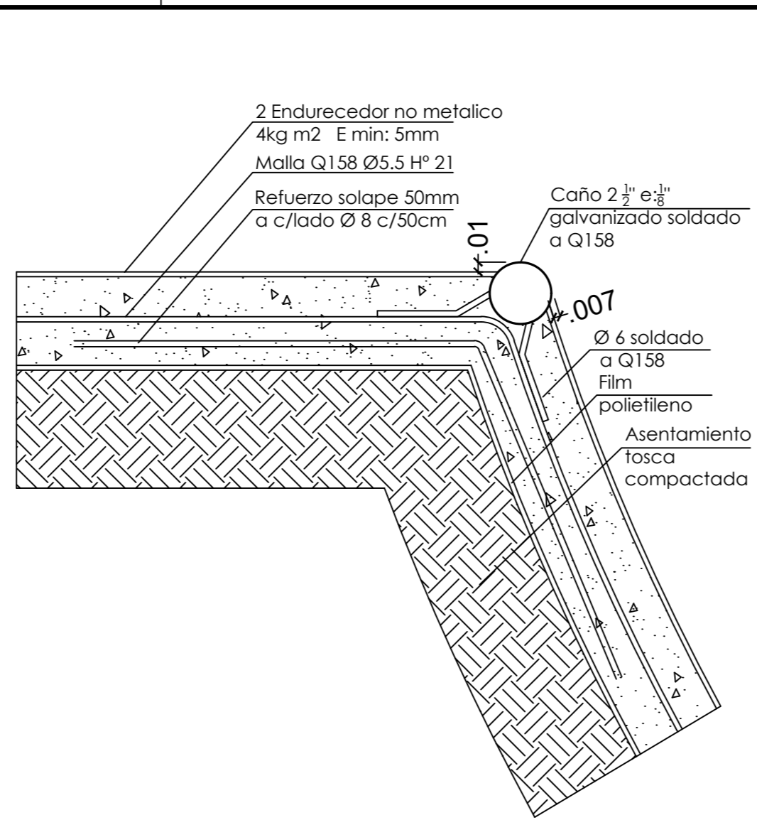
DT02 -Detalle típico de bowl esc. 1:5
