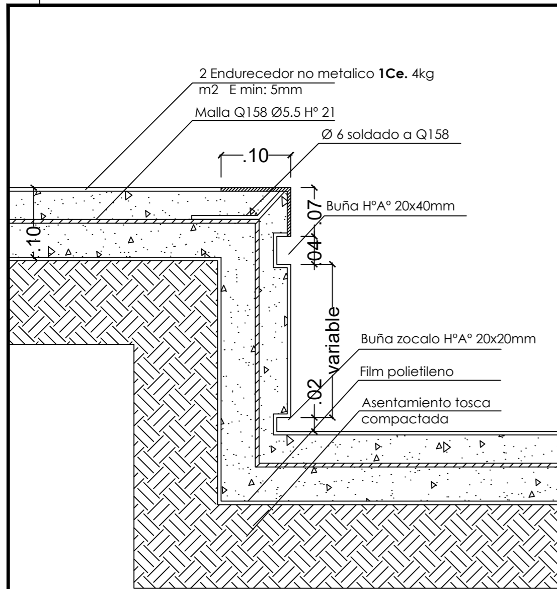
DT01 -Detalle típico de cajon esc. 1:5
