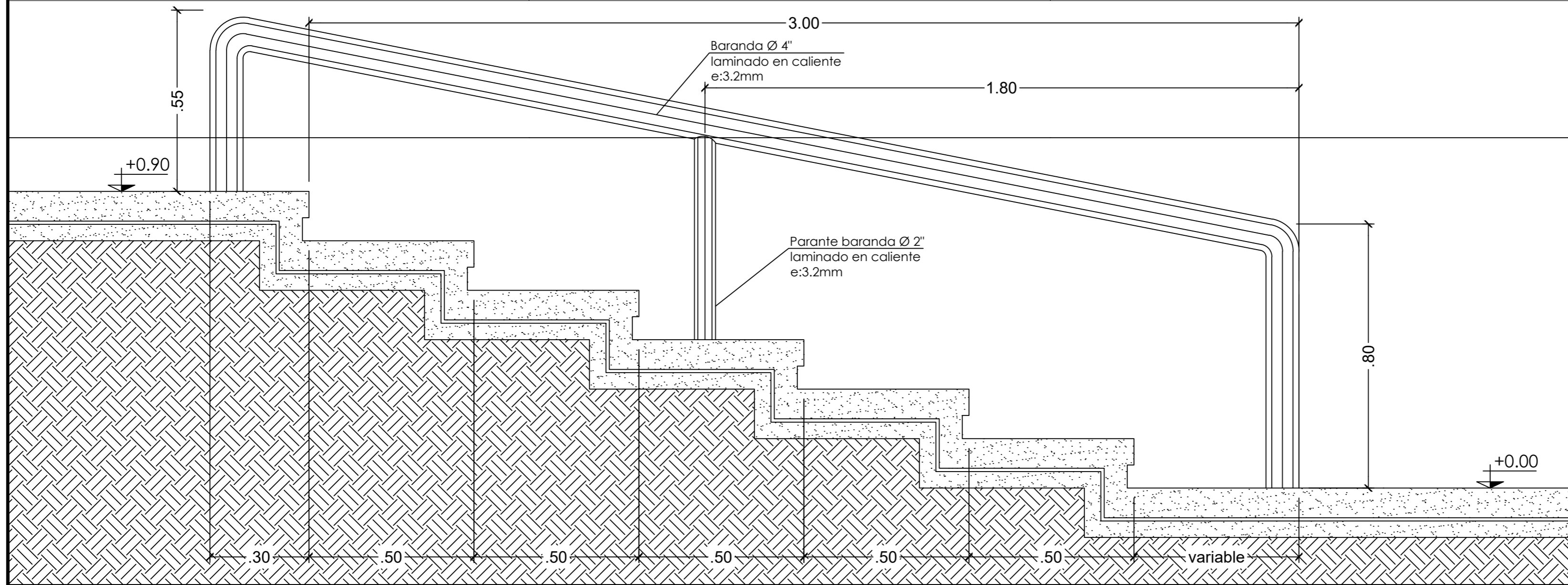
DT04 -Detalle de baranda esc. 1:10
