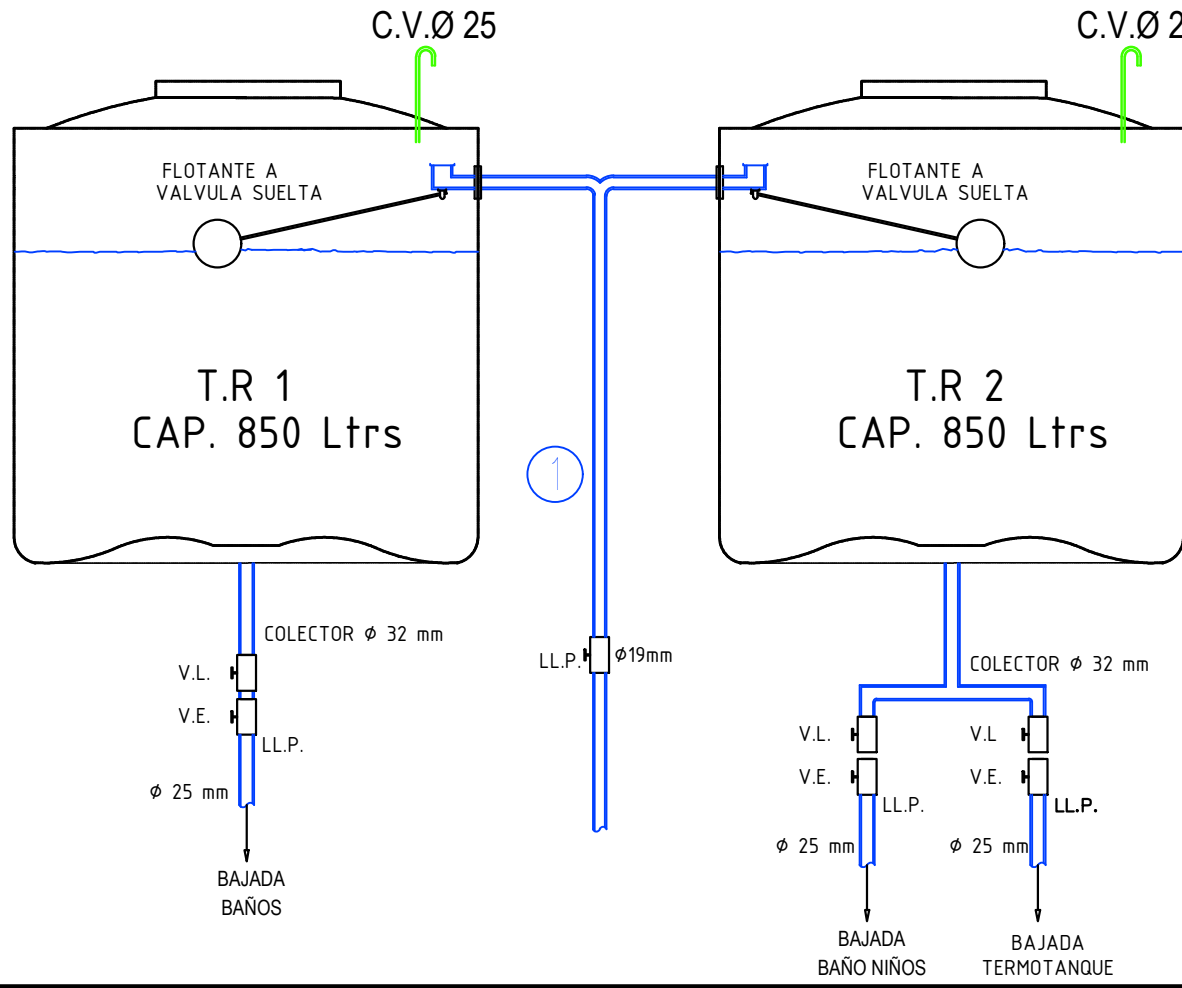
DETALLE COLECTOR T.R.1
